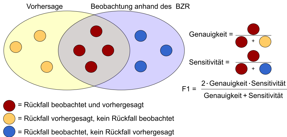
Abbildung 2: Evaluationskriterien für die Vorhersagen von „Rückfall“
