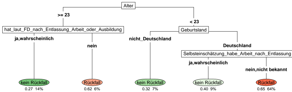
Abbildung 1: Beispiel eines Entscheidungsbaums
